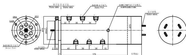
DAIPH600-03 尺寸图
