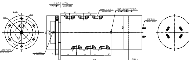
DAIPH600-03 尺寸图
