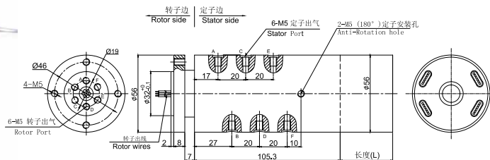
DAIPH600-02 尺寸图
