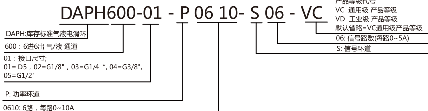
6进6出, D5接头
