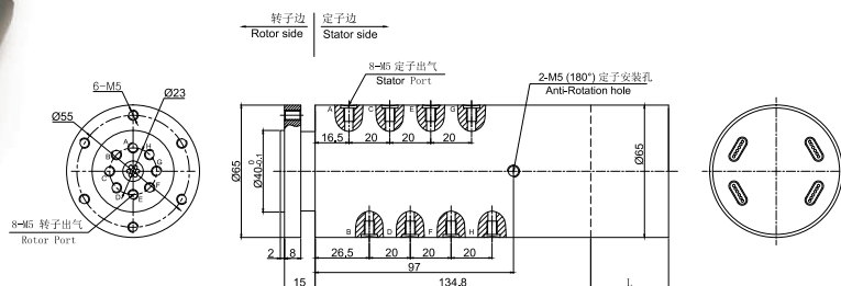
DAPH800-02 尺寸图
