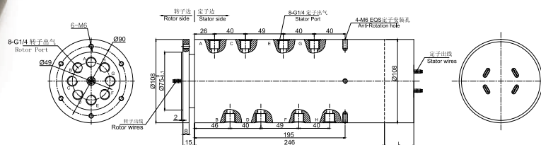
DAPH800-03 尺寸图
