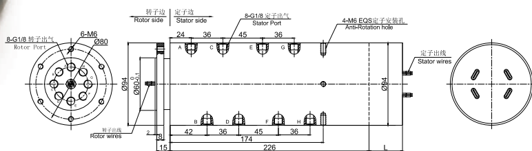
DAPH800-03 尺寸图
